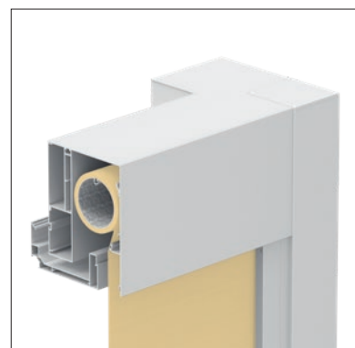
Perfekte Integration der Tuchwelle in die Struktur der VENTUR
